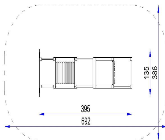
Rzut i widok urządzenia wraz ze strefą funkcjonalną
